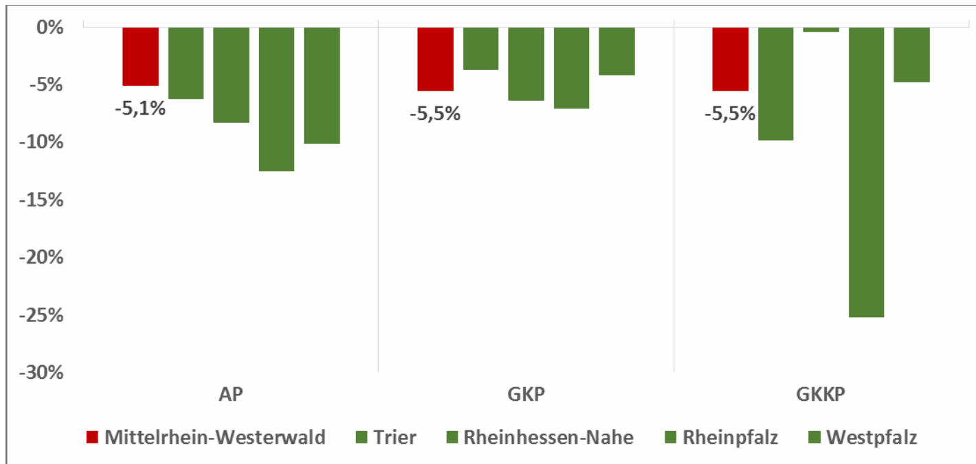
Relative Salden (Saldo / Beschäftigte) für das Jahr 2015
